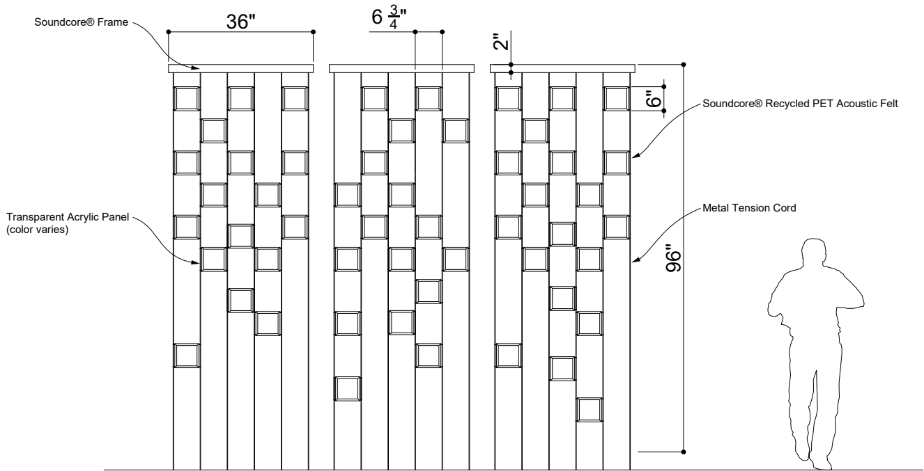
② ELEVATION 2
